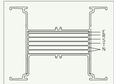
[4W(200%N) + 50%E]
